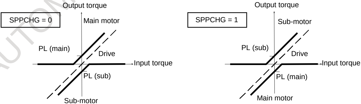
Fig. 4.17.7 (d) Torque output polarity switching and signs of preload values (PL)
