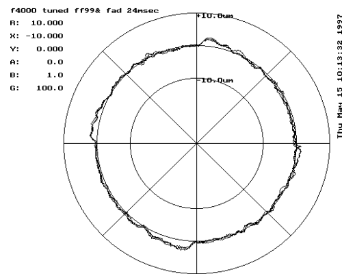
Fig. 3.4.3 (d) Effect of velocity loop gain
