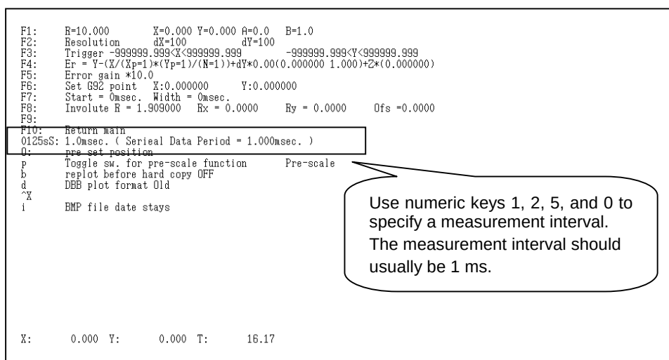
Fig. 4.19 (g) Parameter setting screen
