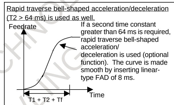
Fig. 3.4.5 (d) Rapid traverse bell-shaped acceleration/deceleration + FAD
