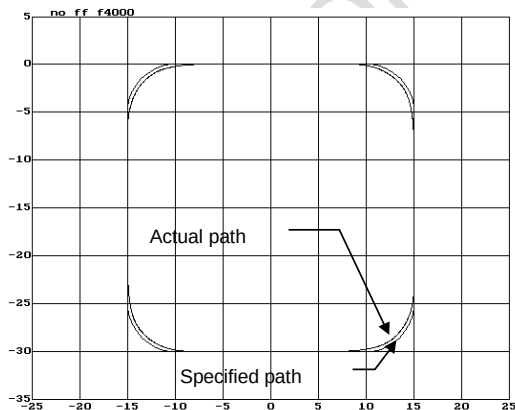
Fig. 3.4.3 (f) Specified path and actual path
