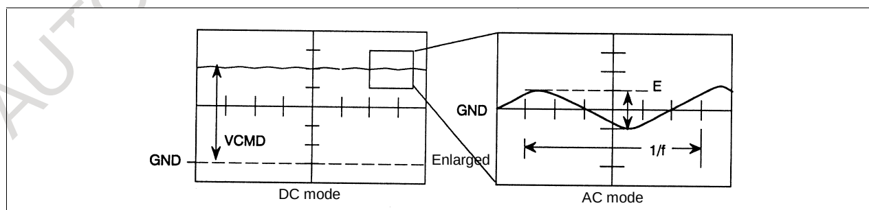
Fig. 4.19 (d) Waveform of the VCMD signal
