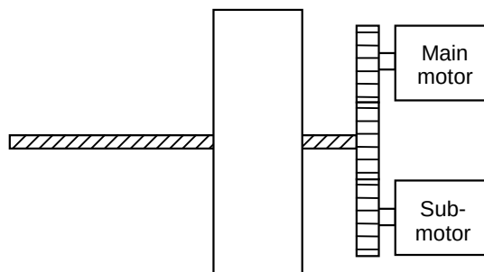
Fig. 4.17.10 (d) Example of tandem control (rigid machine system)
