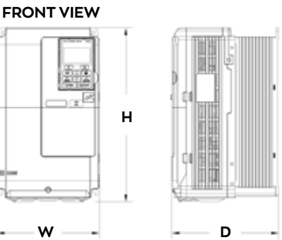
D1000 Dimensions
